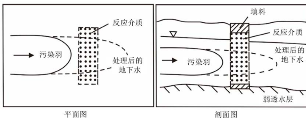
图3-1 连续型PRB示意图
