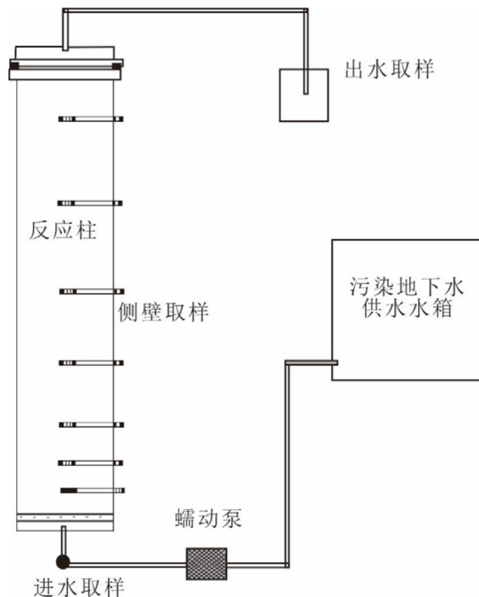
图 5-1 柱实验装置示意图
