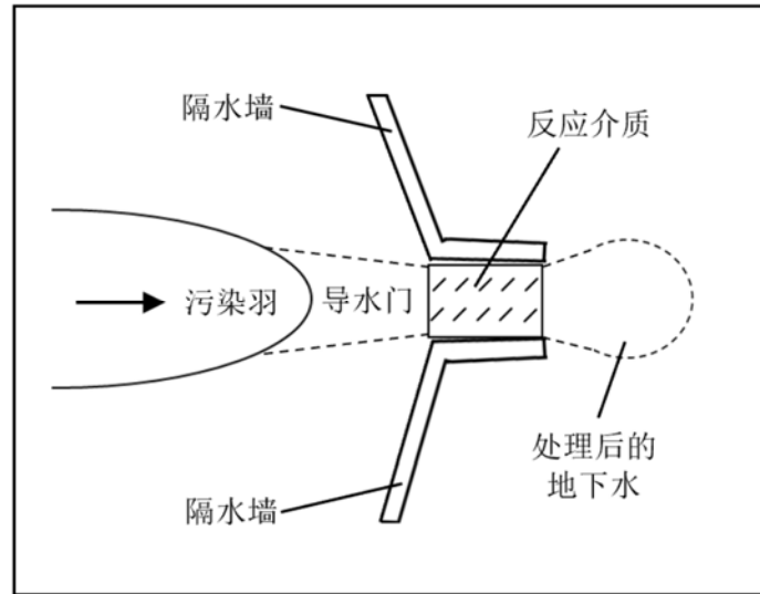
图3-2 漏斗—导水门型PRB示意图
